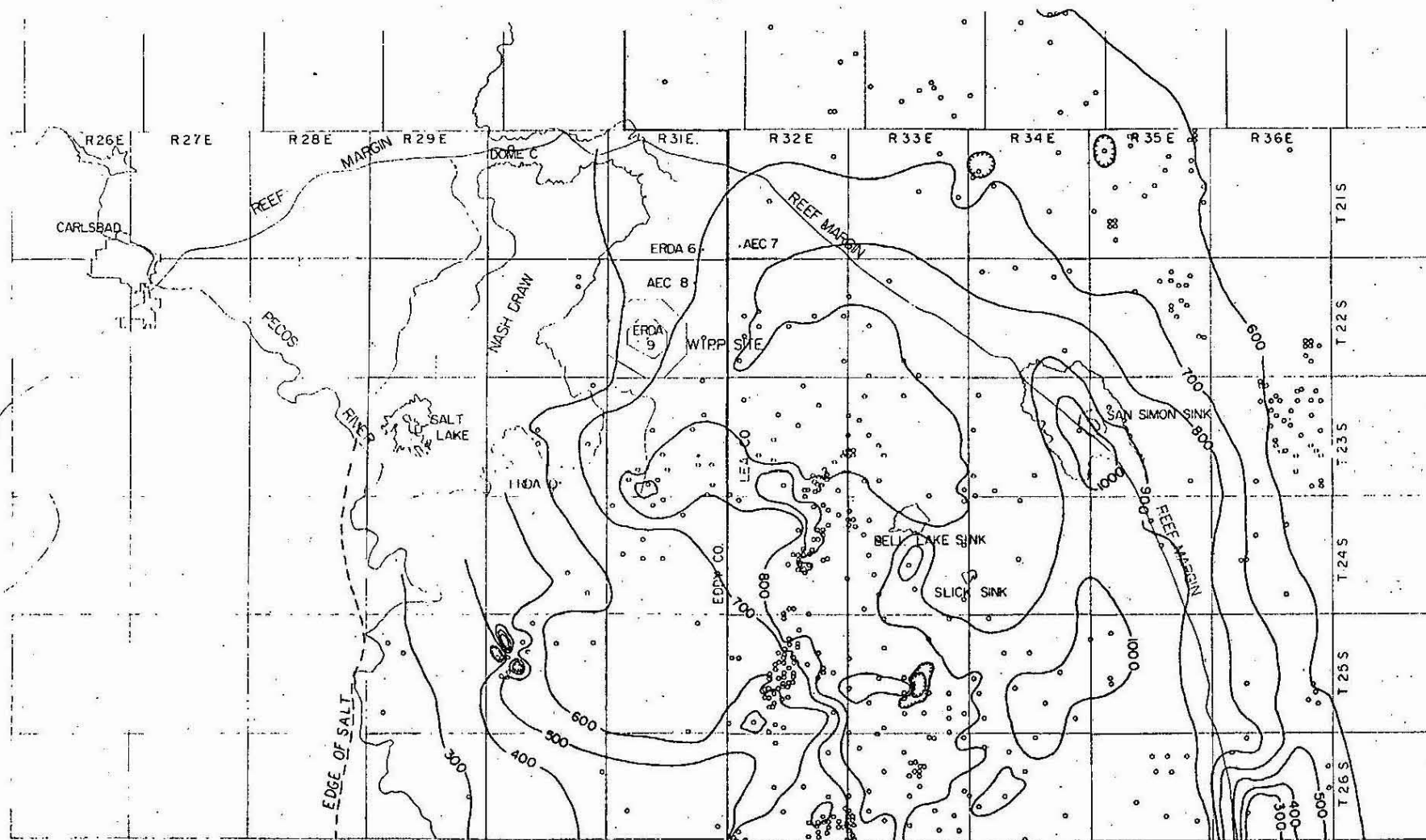
FIG 10 UPPER SALADO ISOPACH
